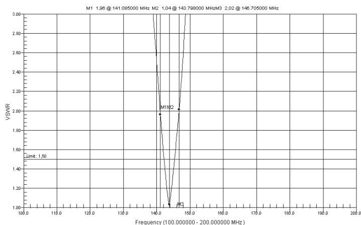
График КСВ в VHF диапазоне
