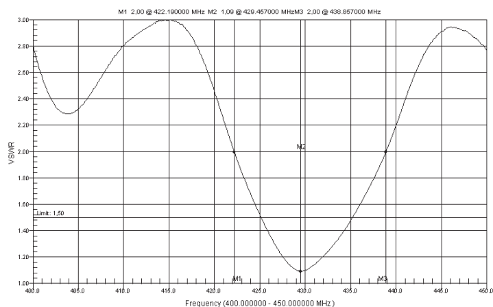
График КСВ в UHF диапазоне
